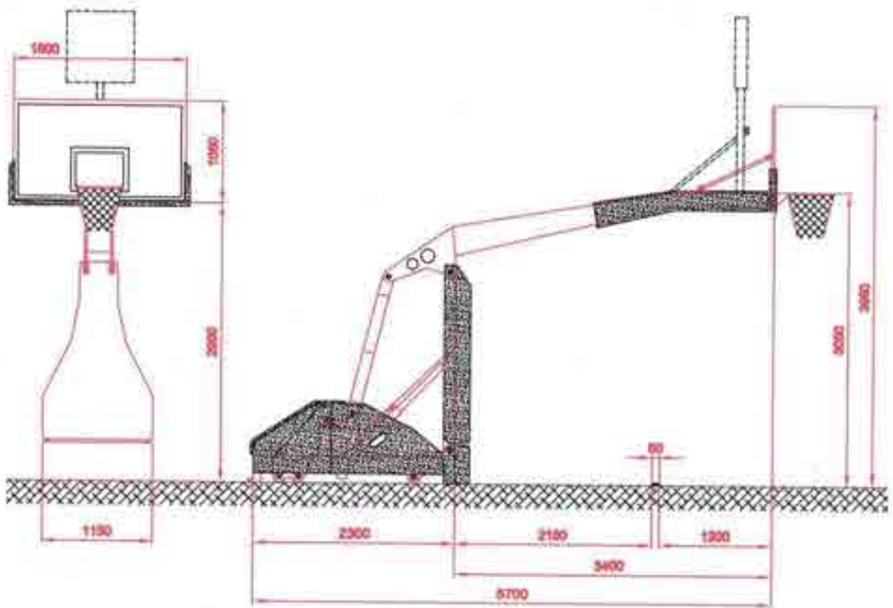
POSIZIONAMENTO IMPIANTO
